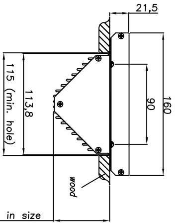
Topview of IR lamppanel (scale 1:5)
